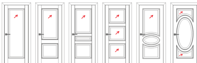
Модель: НЕАПОЛЬ Профили: Тип 1, 2, 3 Размеры Ш: 400-1000 Размеры В: 1900-2400 Модель: ВЕНЕЦИЯ Профили: Тип 1, 2, 3 Размеры Ш: 400-1000 Размеры В: 1900-2400 Модель: АМПИР Профили: Тип 1, 2, 3 Размеры Ш: 400-1000 Размеры В: 1900-2400 Модель: ГРАНД Профили: Тип 1, 2, 3 Размеры Ш: 400-1000 Размеры В: 1900-2400 Модель: ПРОВАНС Профили: Тип 1, 2 Размеры Ш: 550-1000 Размеры В: 1900-2400 Модель: ЛУВР Профили: Тип 1, 2 Размеры Ш: 550-1000 Размеры В: 1900-2400
